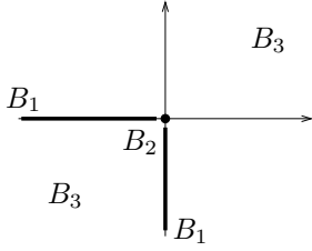
Fig. 5: Suf( \mathcal{P} )
