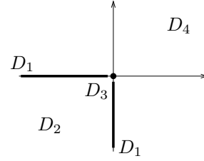
Fig. 7: Suf 3 ( \mathcal{P} )
